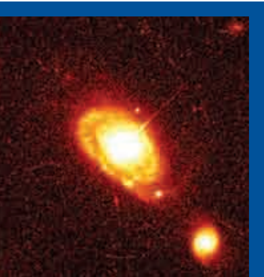
Figura 37.4. Lejano. El cuásar PG 0052+251, a 1400 millones de años luz, en el centro de una galaxia espiral. Fuente: HST.
