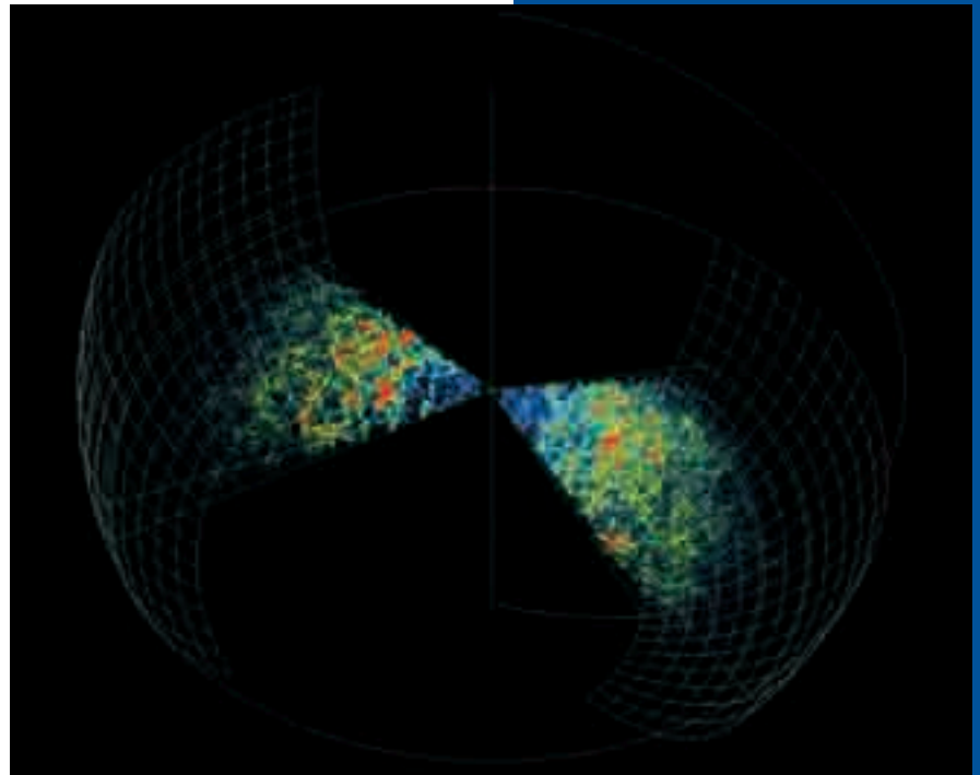
Figura 47.3. Mapa. Distribución en tres dimensiones de galaxias obtenida a partir de los datos del proyecto 2dF.
