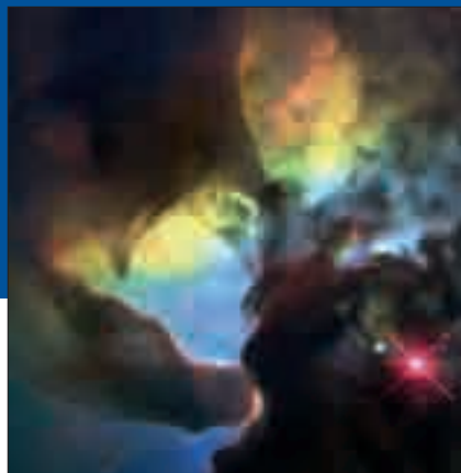
Figura 31.3. Retorcidos. Esta imagen del Telescopio Espacial Hubble (HST) muestra un par de remolinos interestelares en el corazón de la nebulosa Messier 8. Fuente: A. Caulet (ST-ECF, ESA) and NASA.
