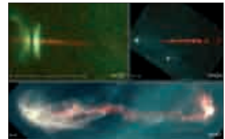
Figura 25.3. Jovencísimas. Arriba a la izquierda vemos la protoestrella HH-30, cuya débil luz ilumina el disco que la rodea, situado de canto. A su derecha observamos la más lejana HH-34, que expulsa gas en forma de chorro a alta velocidad. La imagen inferior muestra a HH-47 (situada en el extremo izquierdo), que presenta un extenso chorro de material eyectado. Fuente: STScI, ESA, Univ. Arizona y NASA.
